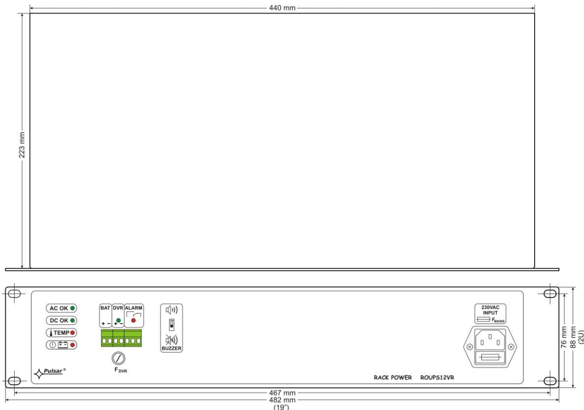
Rys.3. Widok zasilacza.
